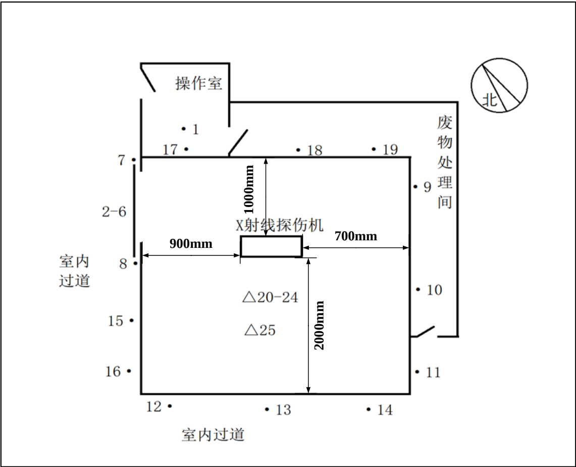
图 11-2 特技阀门集团有限公司 X 射线探伤室监测点位示意图
