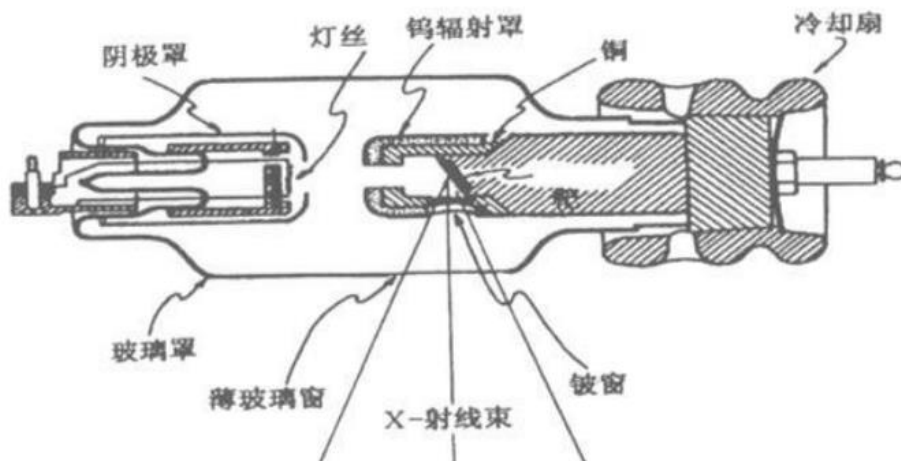
图 9-3 典型 X 射线管结构图
