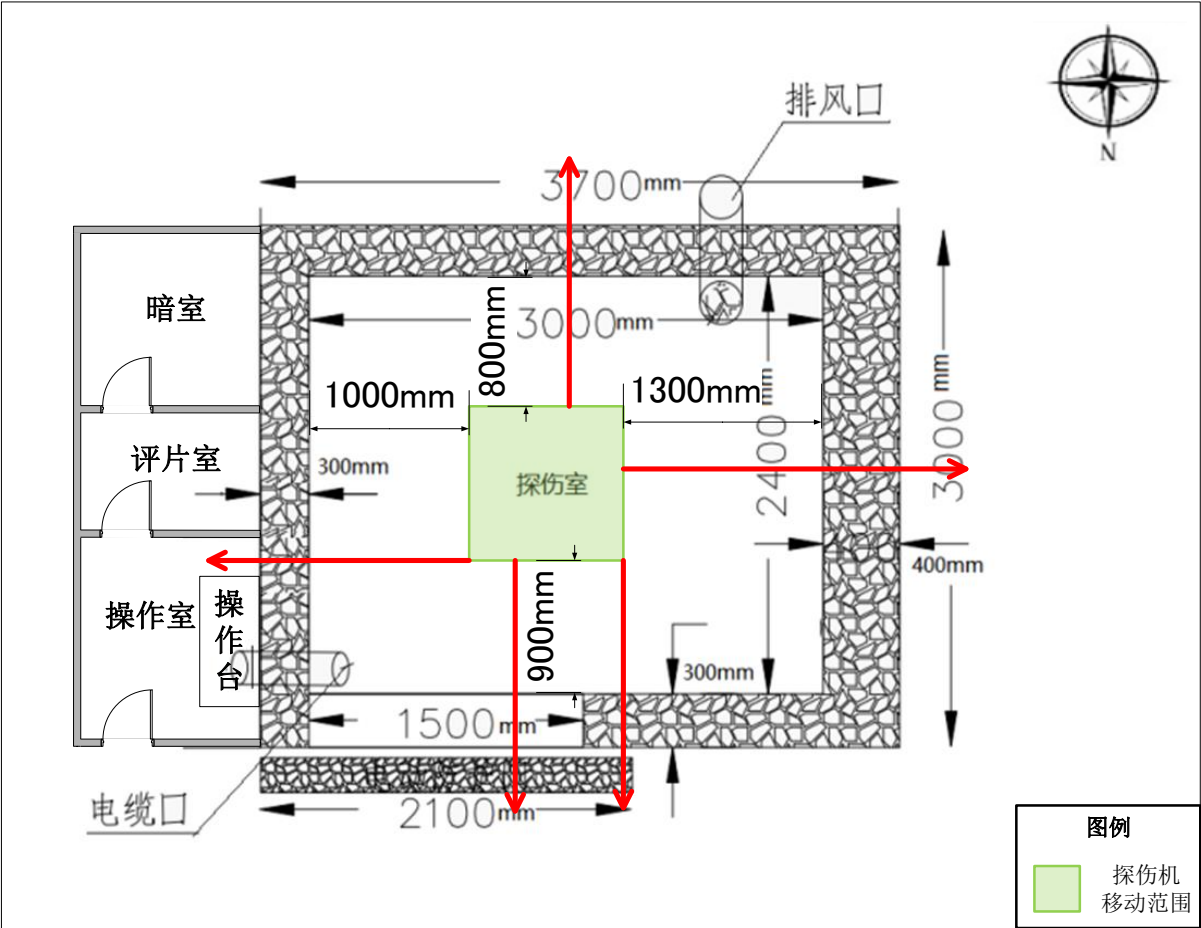
图 11-1 屏蔽计算预测点位图
